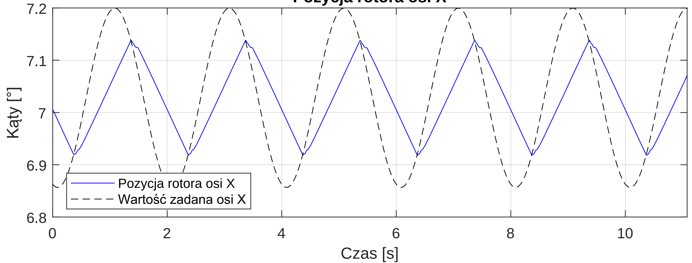
Pozycja rotora osi X
