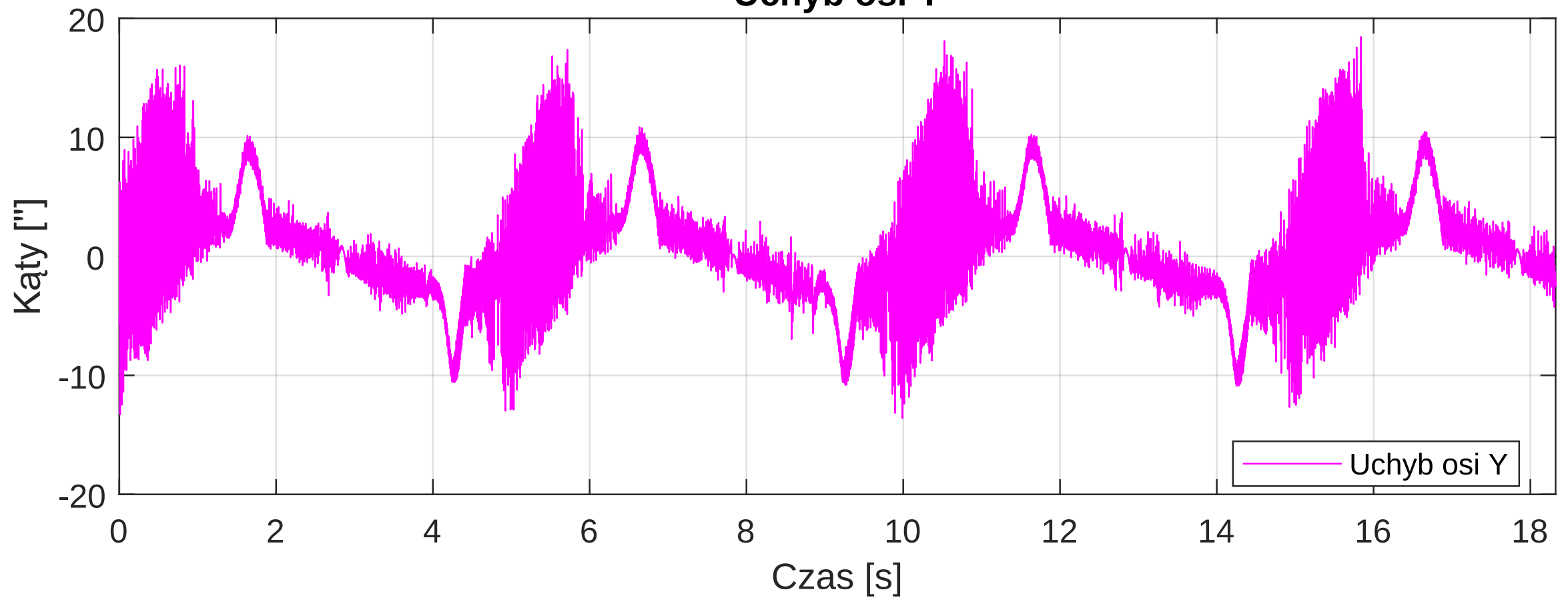
Uchyb osi Y
