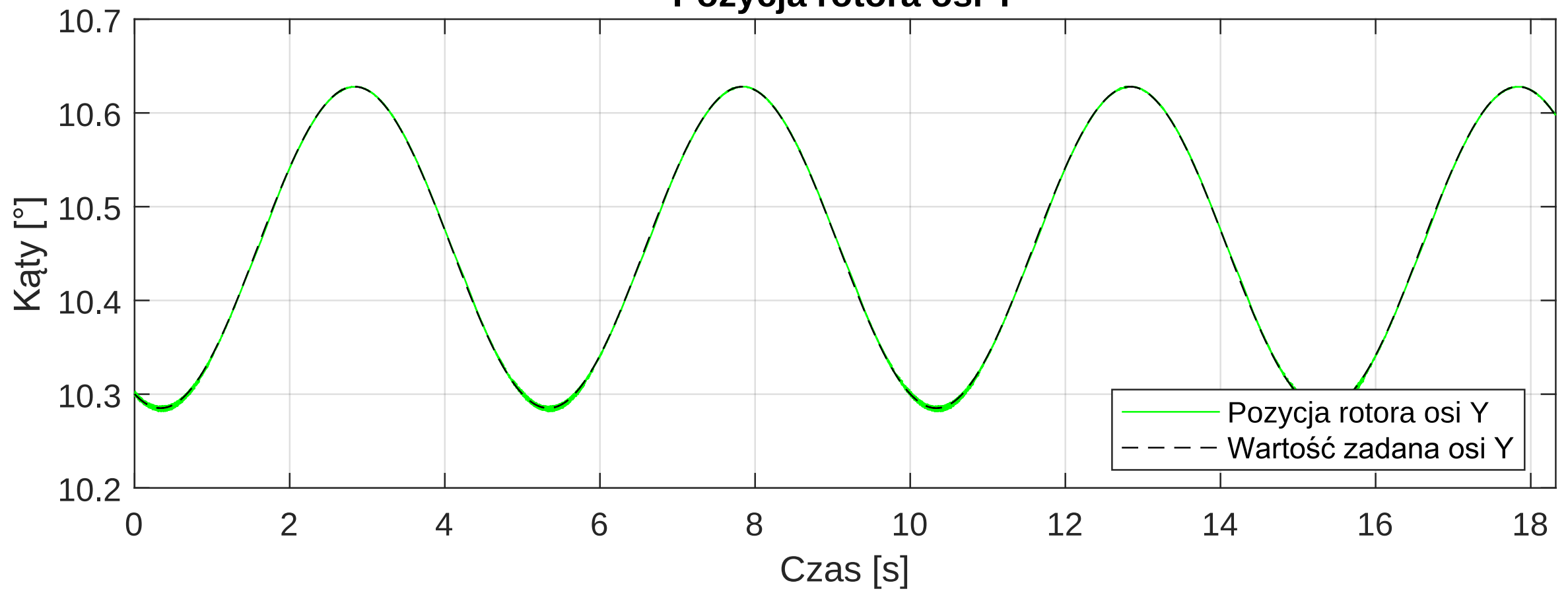
Pozycja rotora osi Y
