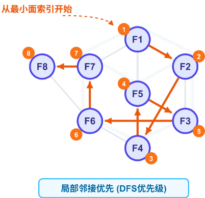
(b) 深度优先排序 (DFS face ordering)
