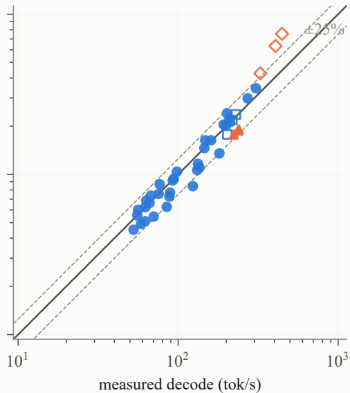
RTX 5080
