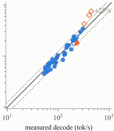
RTX 5080
