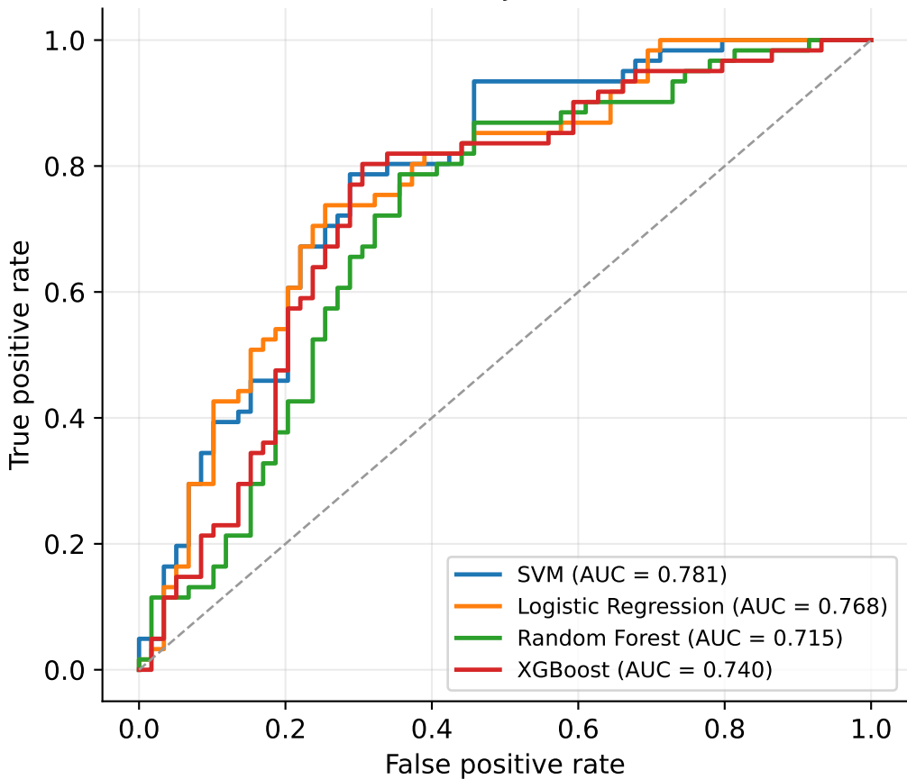
ROC curves (subject-level, LOSO)
