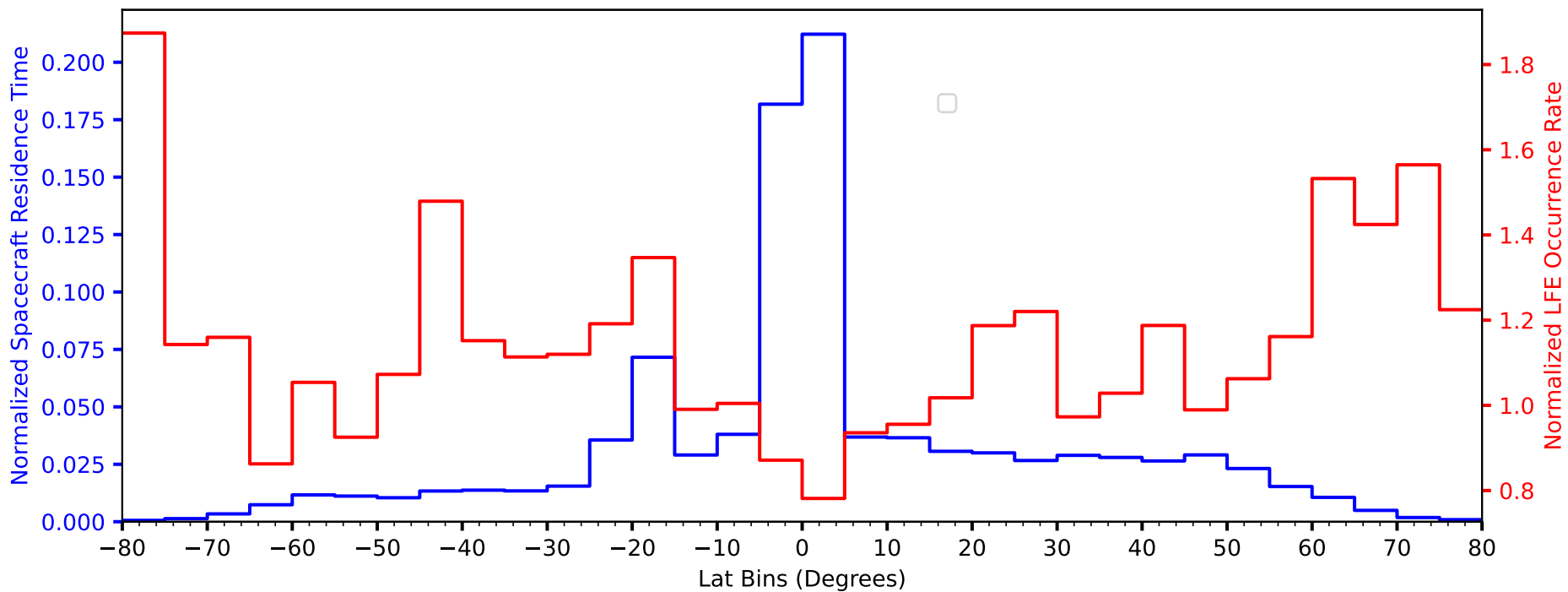
Latitude (Lat) Distribution of LFEs
