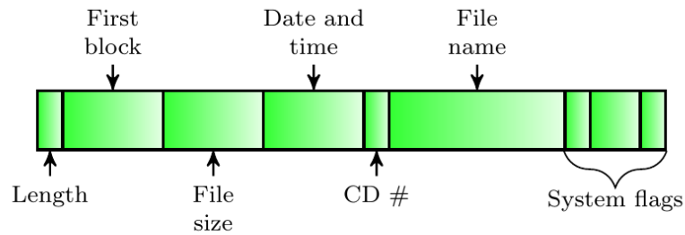
Entrada de directorio en ISO-9660 (CD-ROM)
