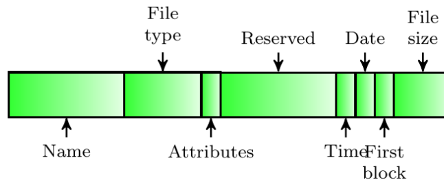
Entrada de directorio en FAT (MS-DOS)
