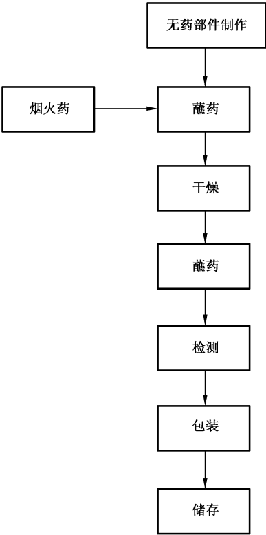
图 A. 22 电点火头生产流程图
