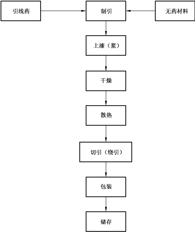
图 A.3 安全(皮纸)引线生产工艺流程图
