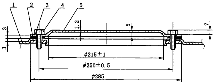
图 A.1 桶顶下部加固封闭器的外形和装配关系
