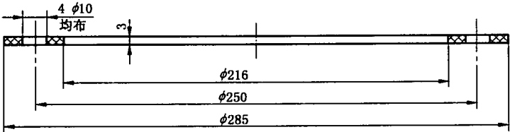
图 A.4 密封圈
