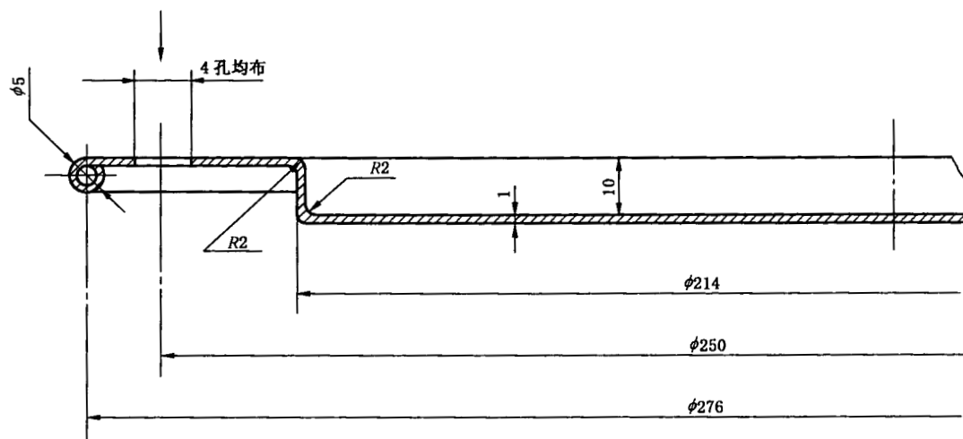
K 向局部视图
