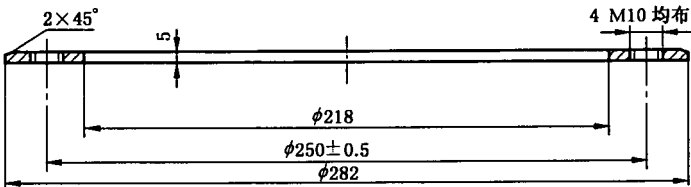
图 A.3 法兰圈
