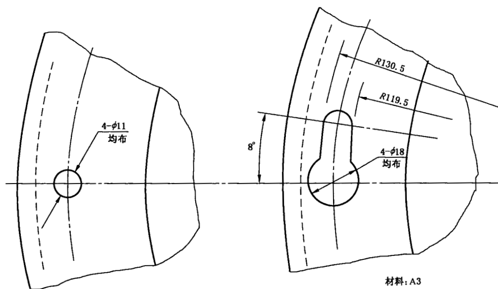
第一种结构圆孔
