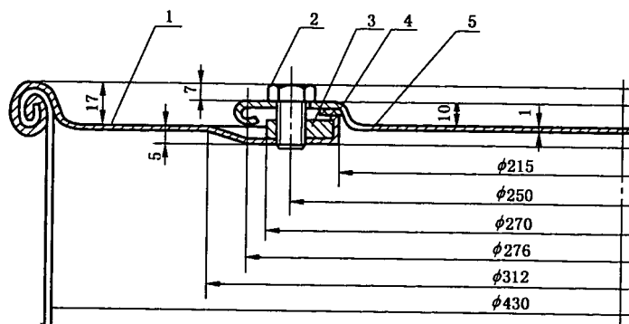
图 A.7 封闭器外形和装配关系(桶顶上部加固)
