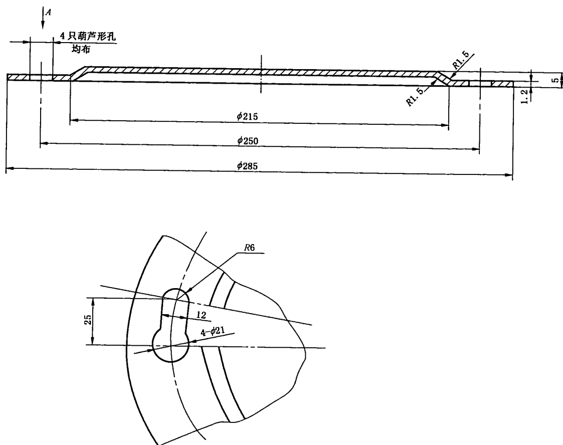
图 A.6 桶盖
