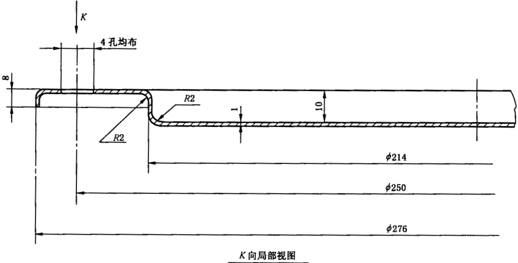
第一种结构圆孔
