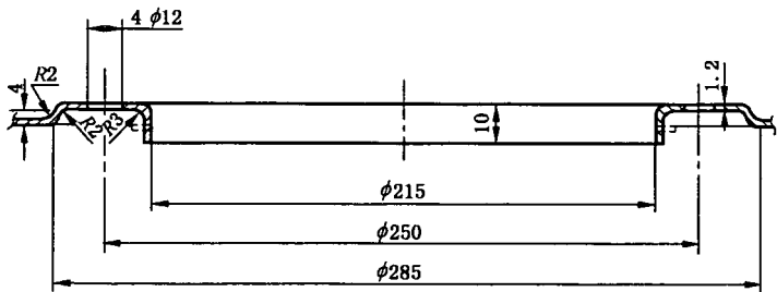
图 A.2 桶口形状和尺寸
