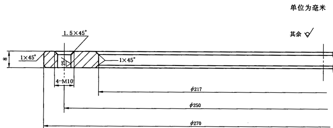
图 A.8 加固圈
