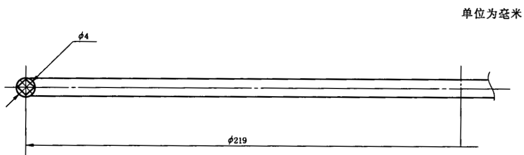
图 A.9 O形密封圈
