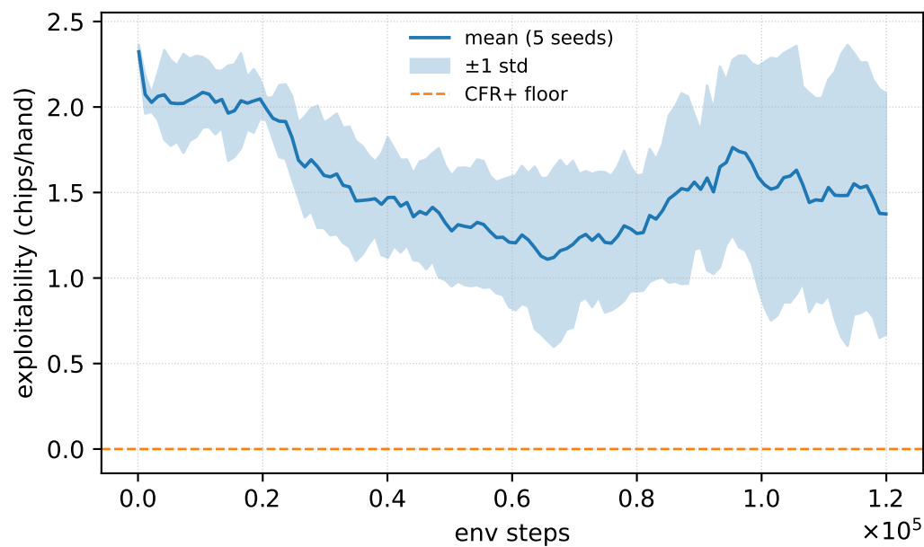
PPO
