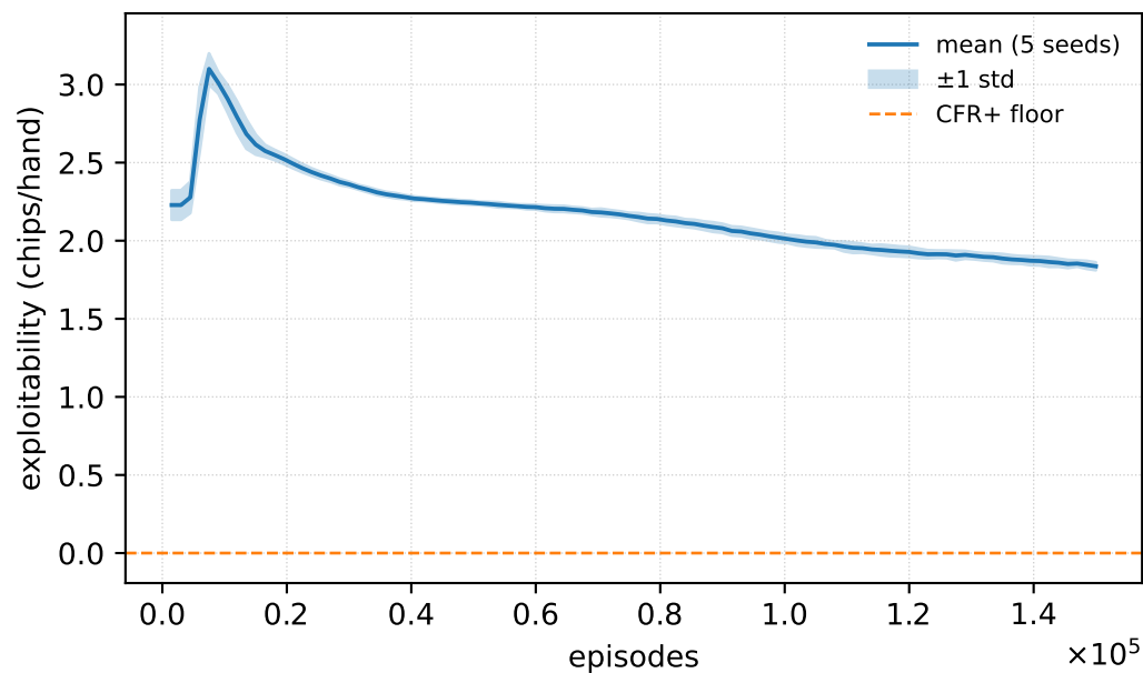
NFSP
