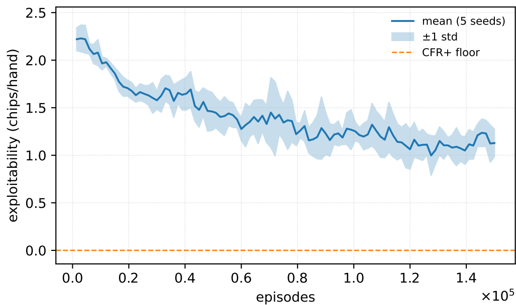
RMPG
