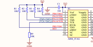
JTAG/SWD调试接口
