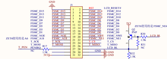
TFT液晶屏接口
