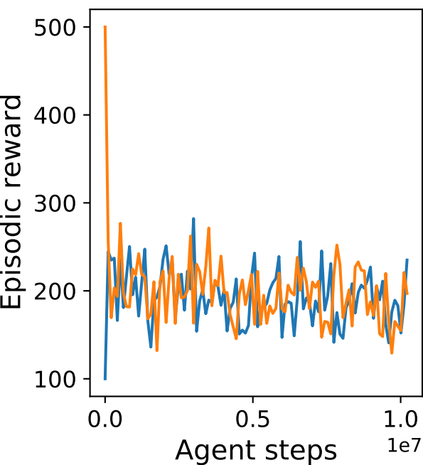
Gravitar
