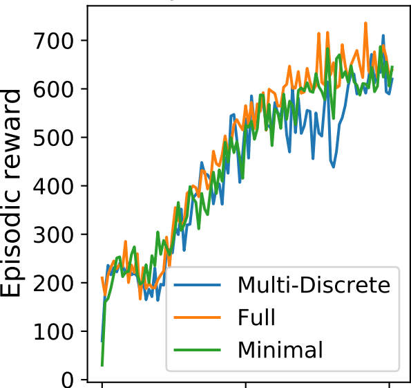
SpaceInvaders
