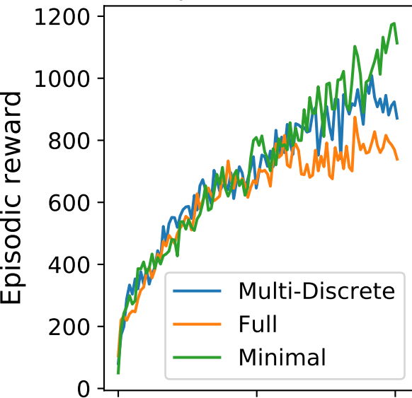
SpaceInvaders
