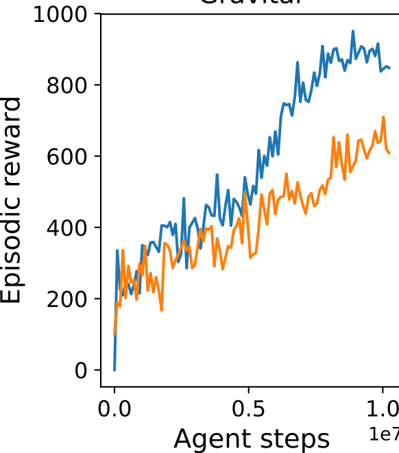
Gravitar
