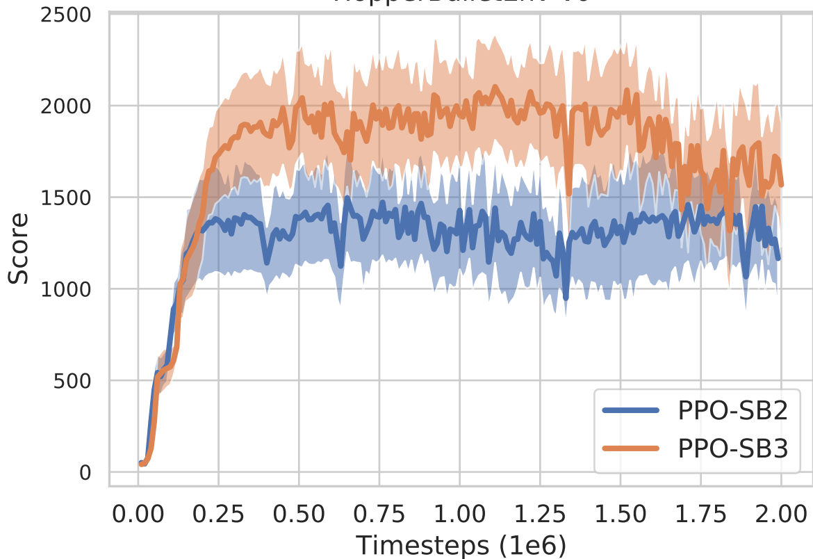
HopperBulletEnv-v0
