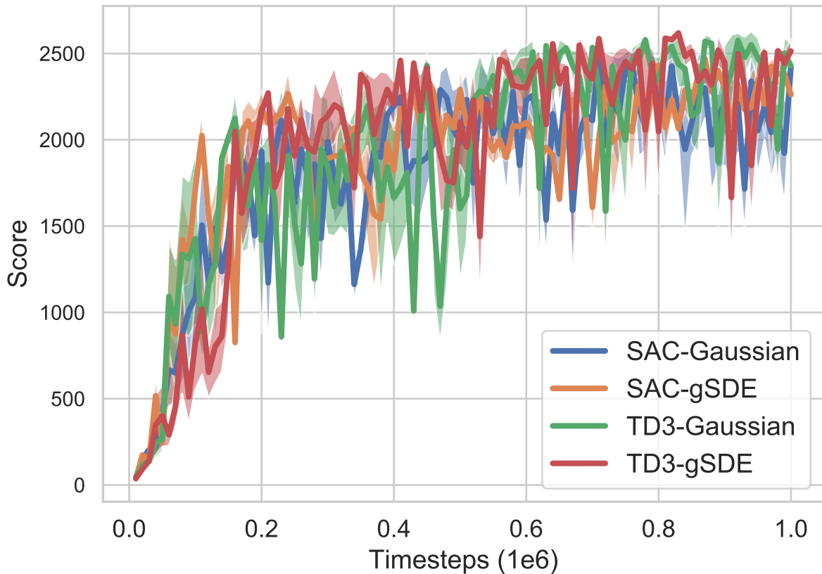
HopperBulletEnv-v0
