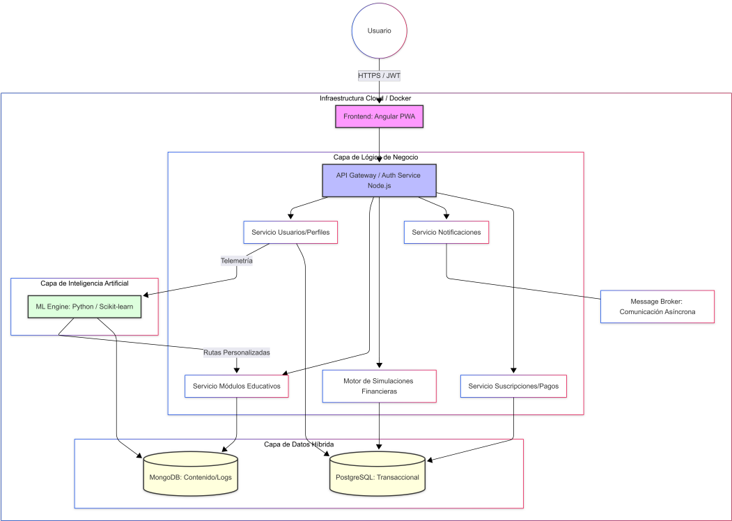
Figura 13: Arquitectura Lógica de Microservicios de la Plataforma.
