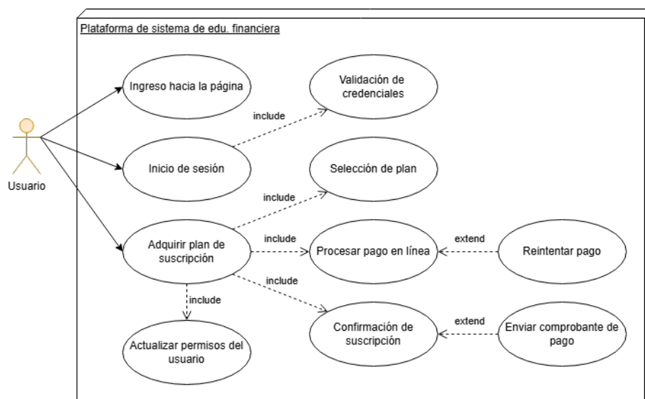
Figura 21: Diagrama de caso de uso RF07. Fuente: Autores.
