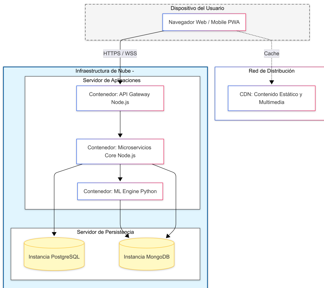
Figura 14: Diagrama de Despliegue de Infraestructura en la Nube.
