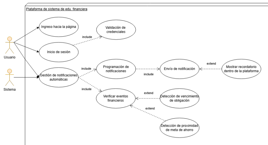
Figura 20: Diagrama de caso de uso RF06. Fuente: Autores.
