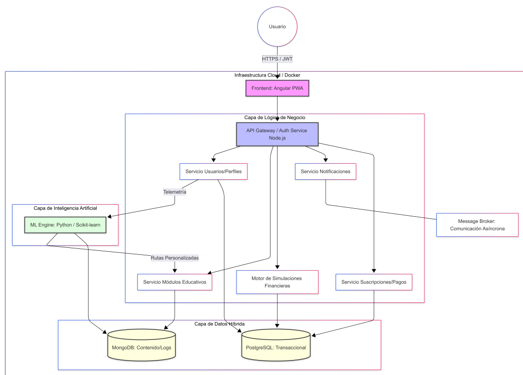
Figura 13: Arquitectura Lógica de Microservicios de la Plataforma.
