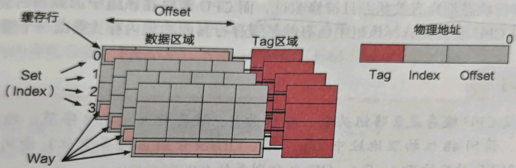
图 5.11 典型的 CPU 缓存结构示意图 [7]
