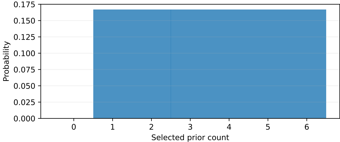
Mask-SC-oracle
