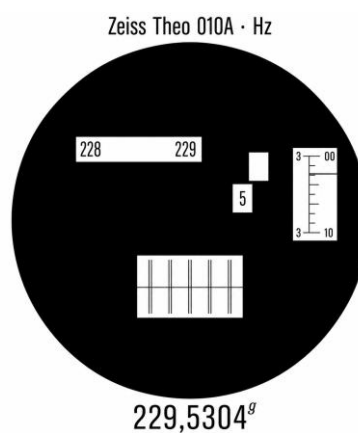
Obr. 2 Zeiss Theo 010A – bod 1003
