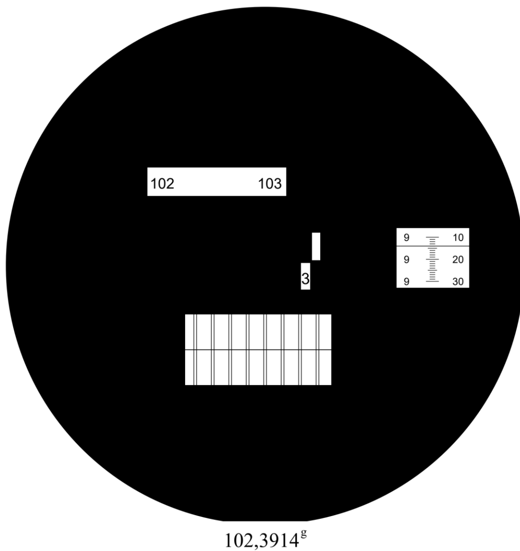
Obr. 2 Zeiss Theo 010A
