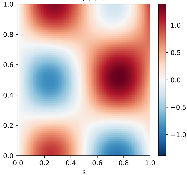
True \beta(s, t)
