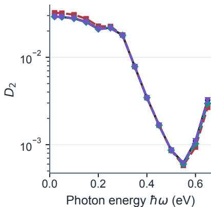
(b) Compact MS-CASPT2
