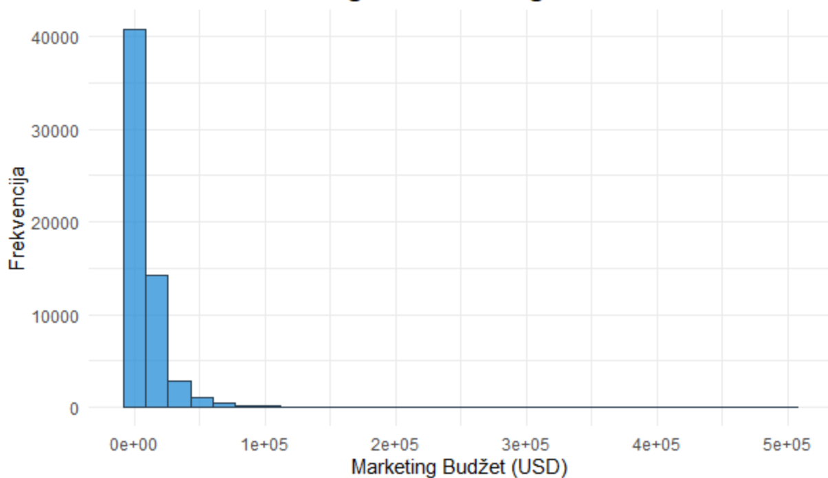
Histogram: Marketing Budžet
