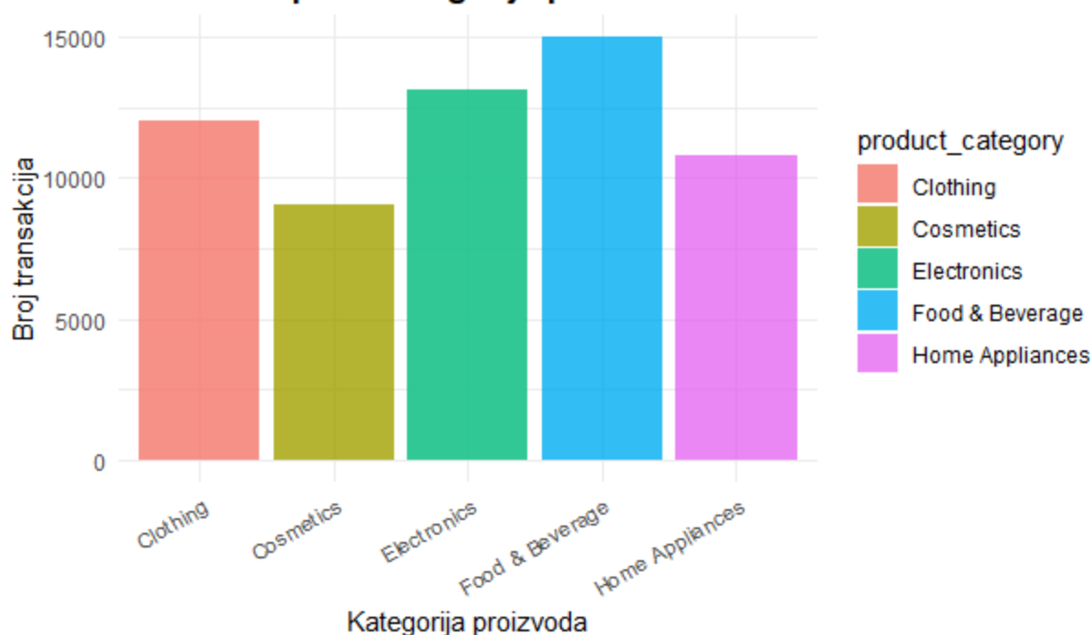
Bar plot: Kategorije proizvoda
