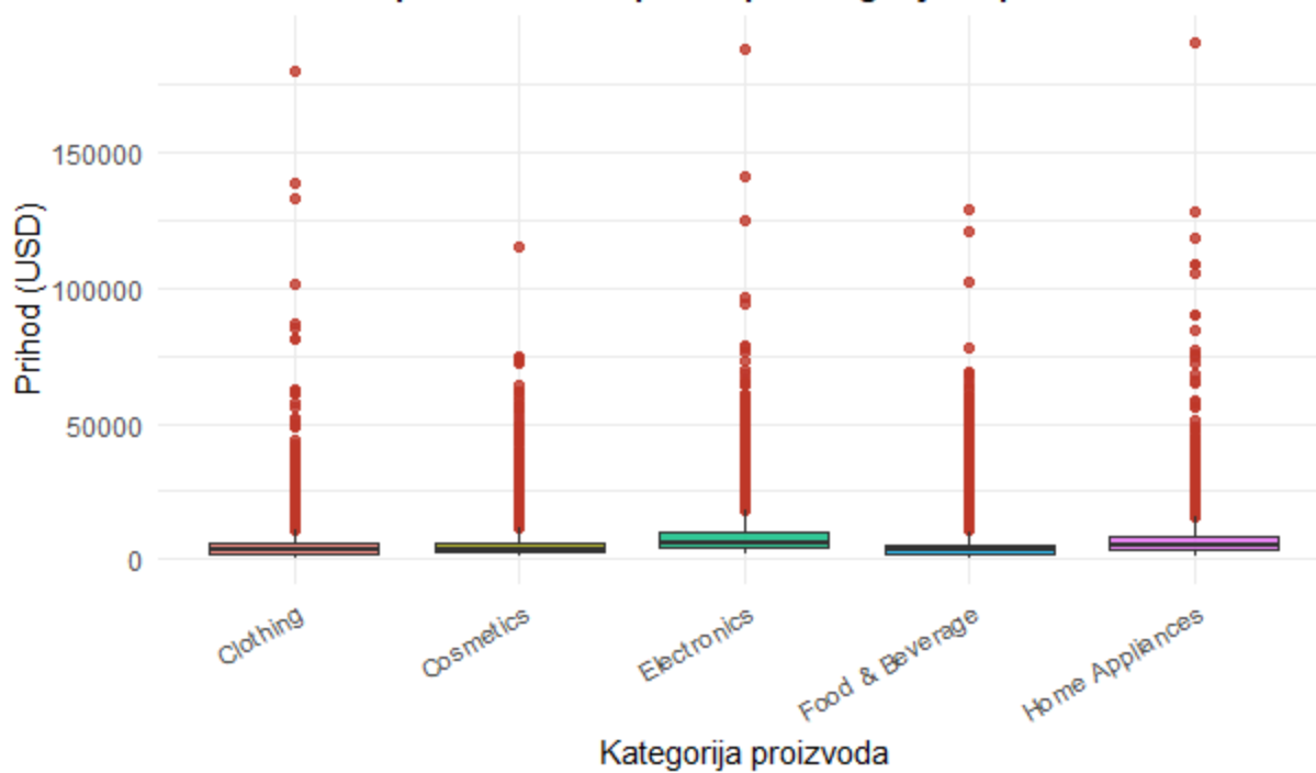
Boxplot: Ostvareni prihod po kategorijama proizvoda
