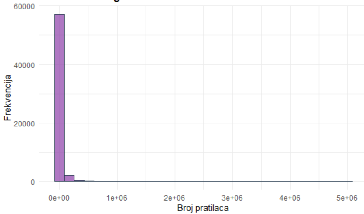
Histogram: Pratioci na društvenim mrežama
