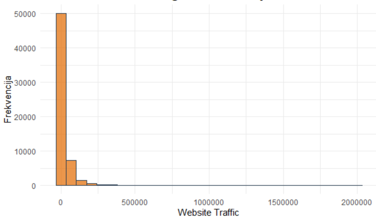
Histogram: Posete sajtu
