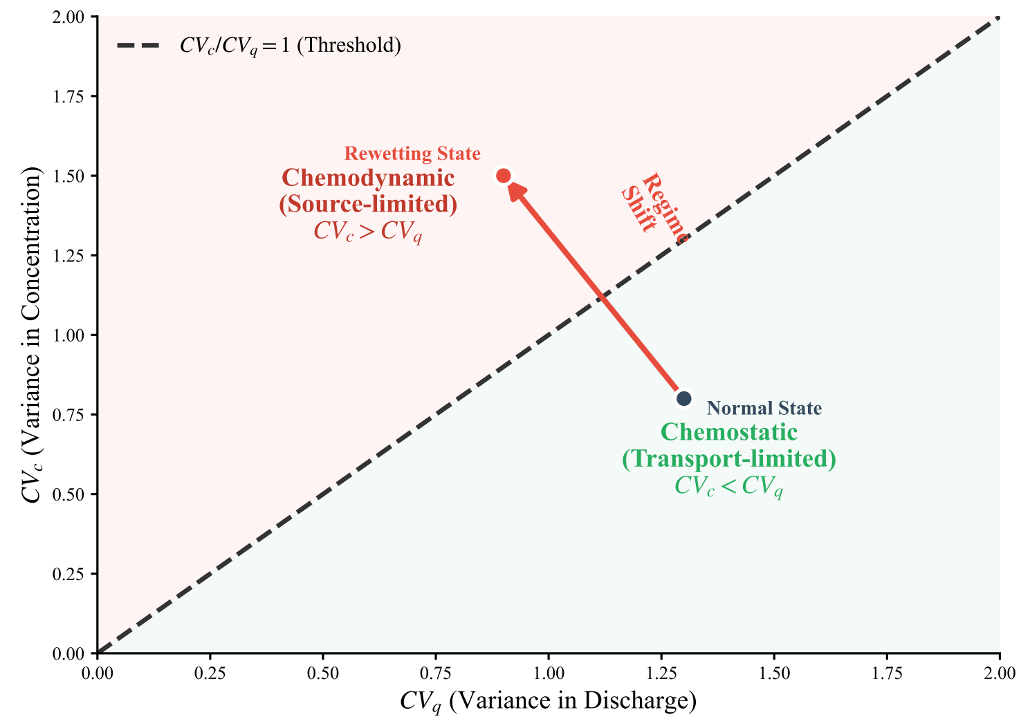
(d) Chemostatic Index ( CV_c/CV_q ) & Regime Shifts
