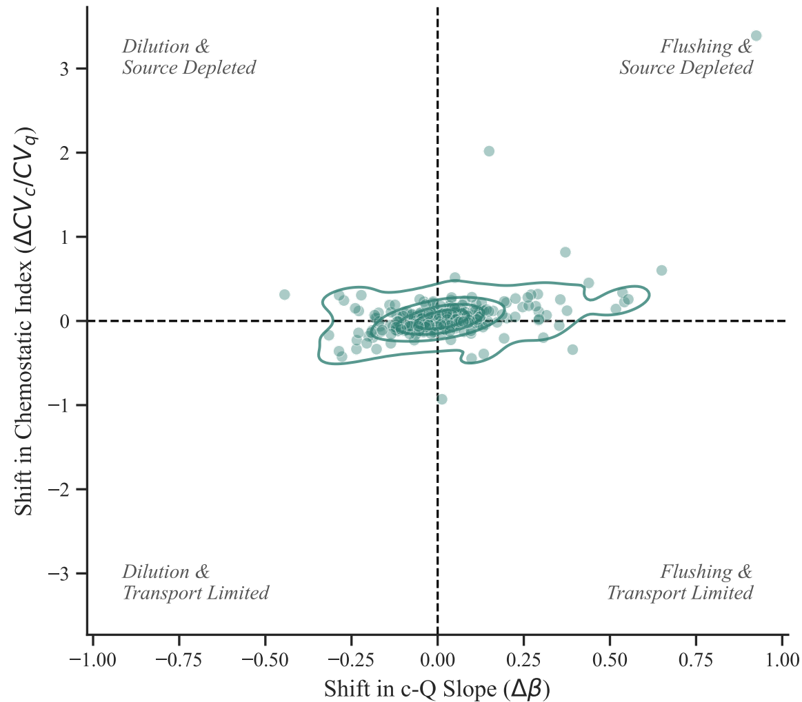
NO3N Regime Shifts
