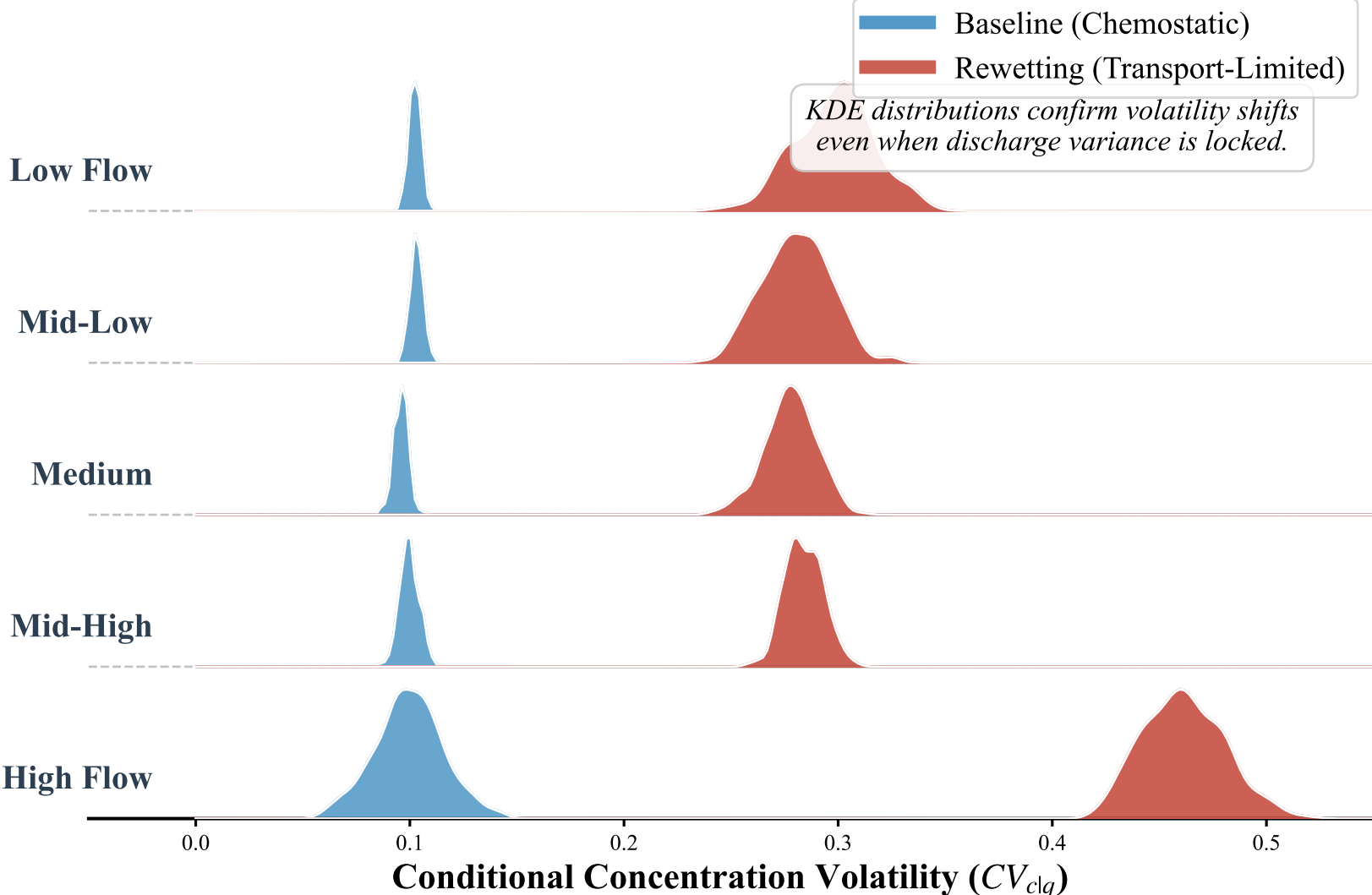
(d) Quantile-Stratified Volatility (Ridge Plot)
