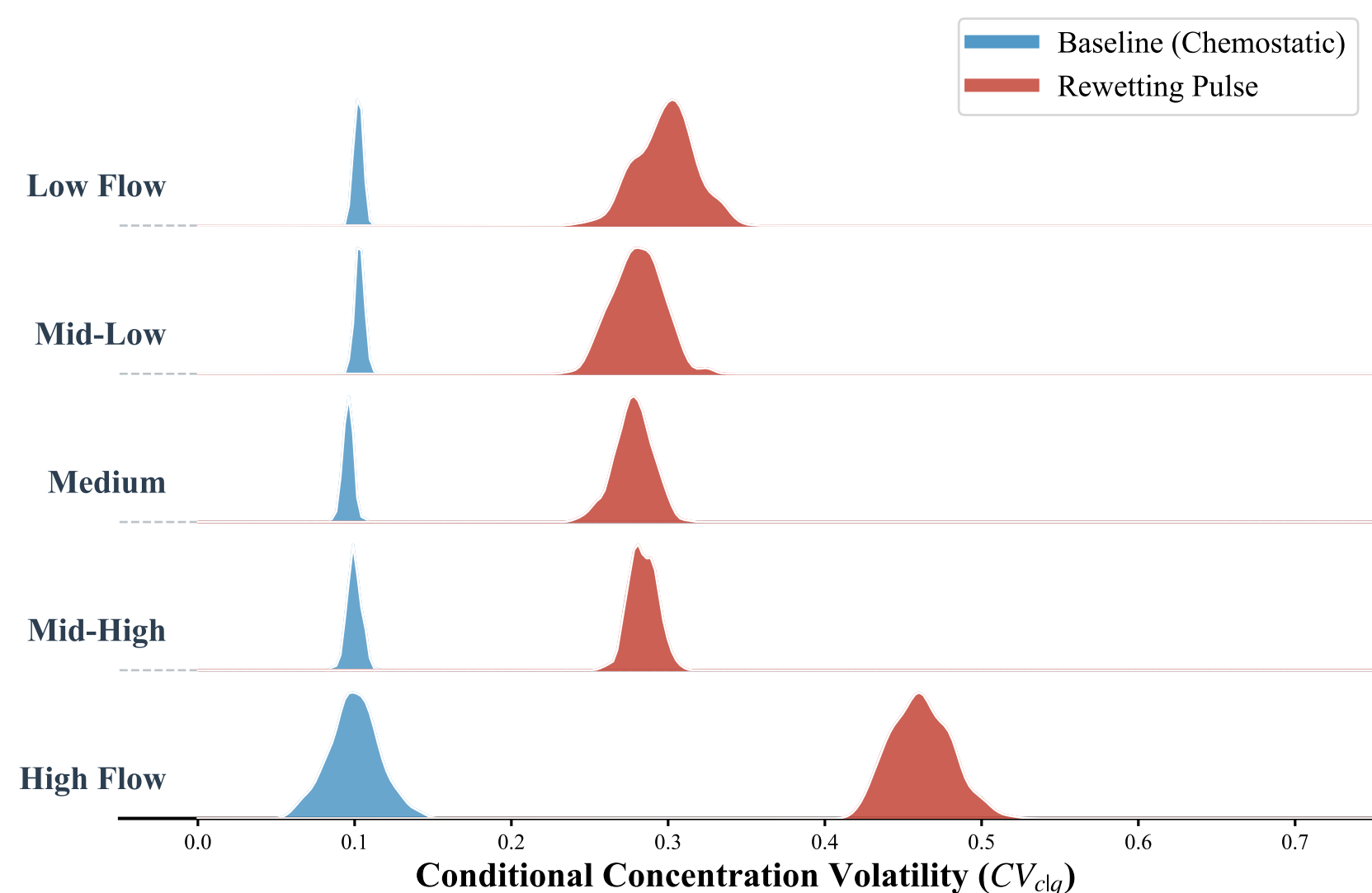
(d) Quantile-Stratified Volatility (Ridge Plot)
