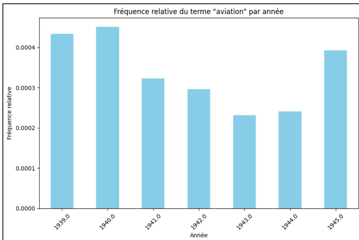
Figure 3 Fréquence relative du terme "aviation" par année
