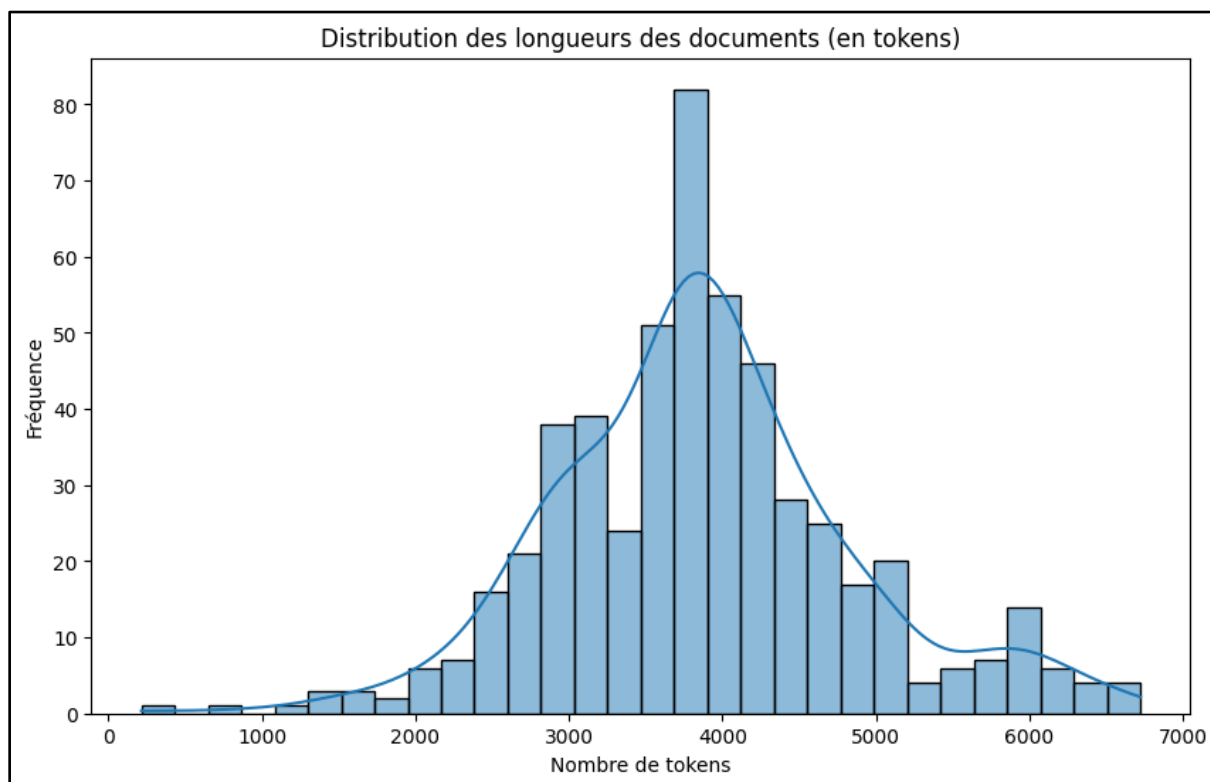
Figure 2 Distribution des longueurs des documents (en tokens)
