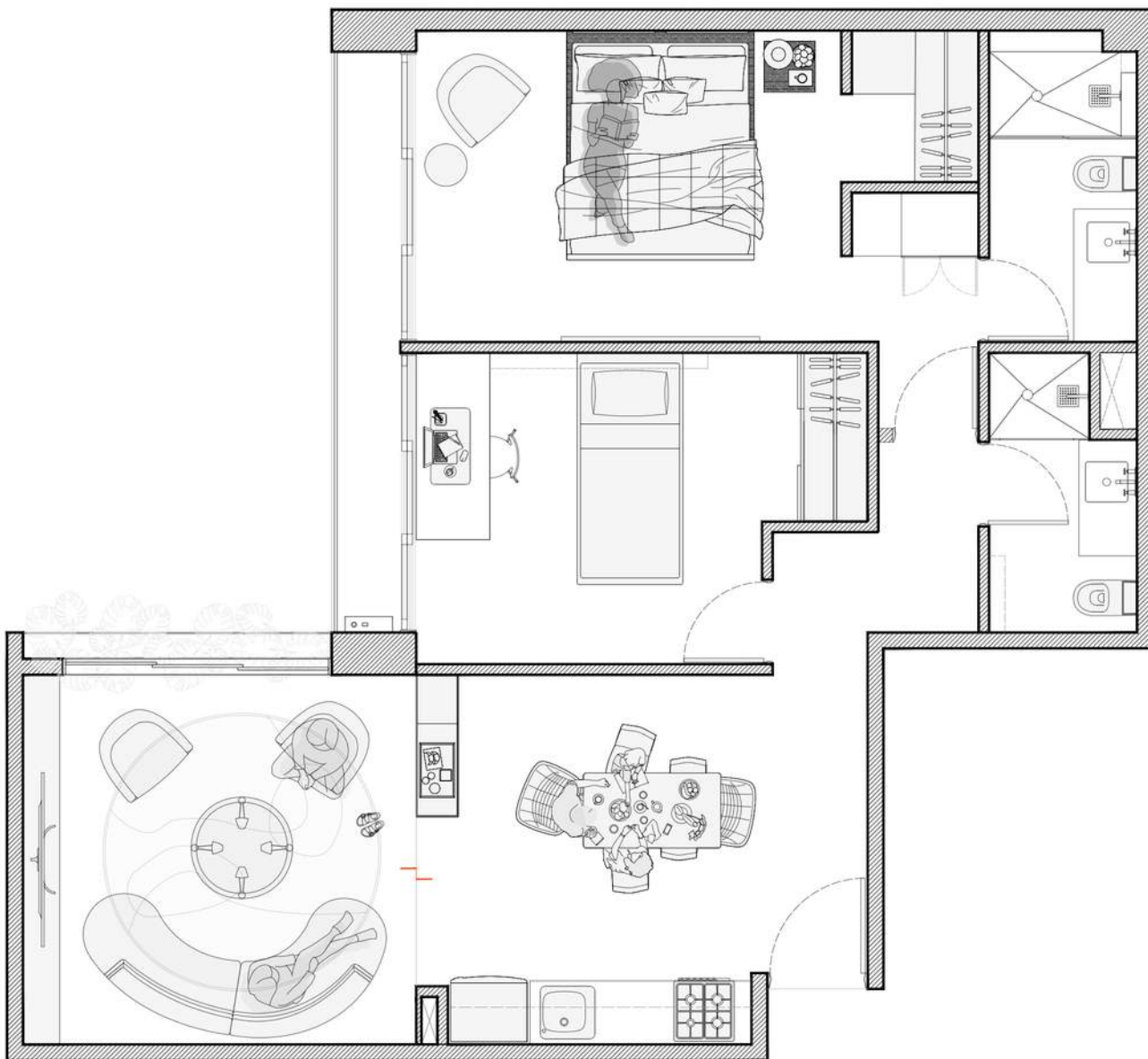
TIPOLOGIA DE DEPARTAMENTO B
