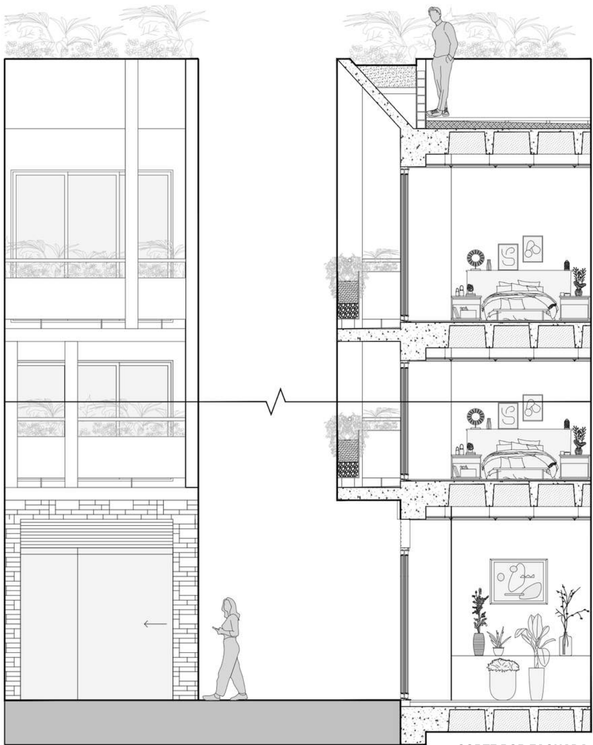
CORTE POR FACHADA
