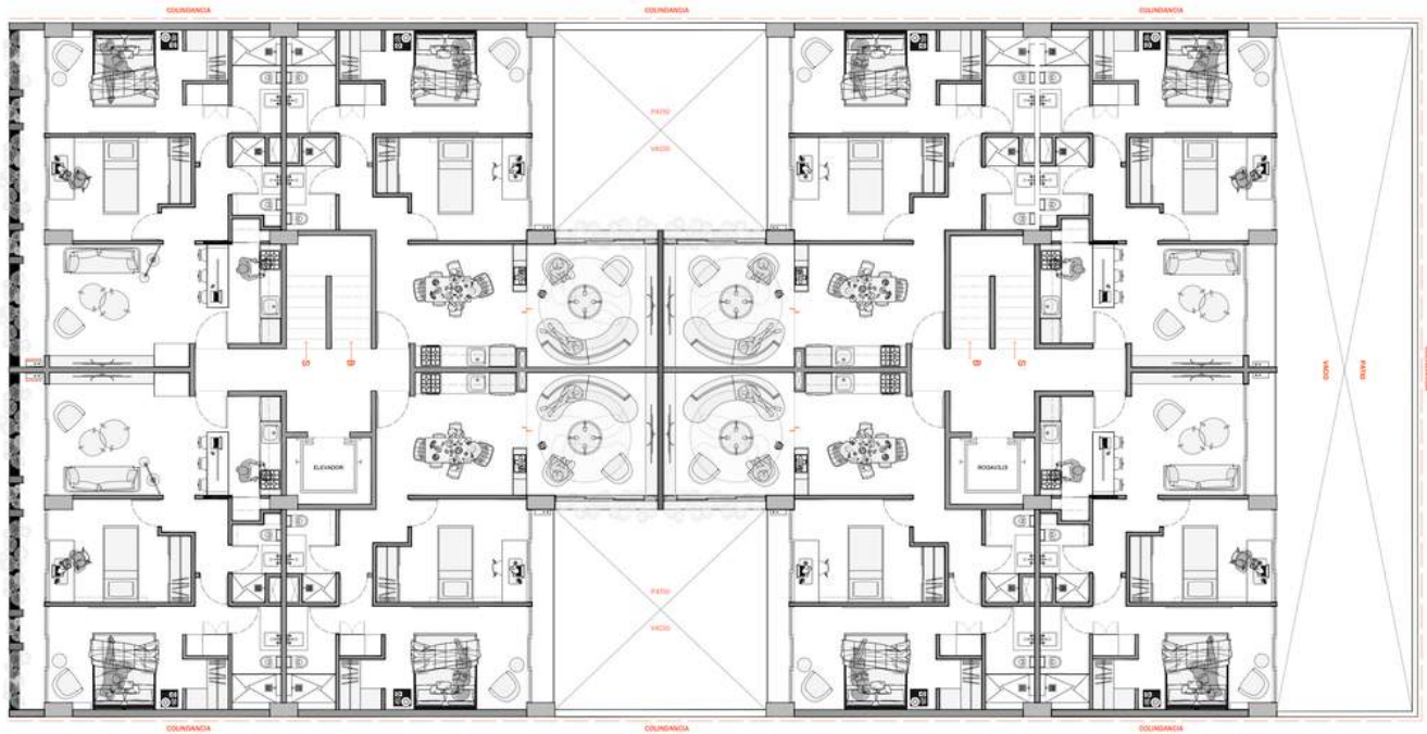
PLANTA TIPO
