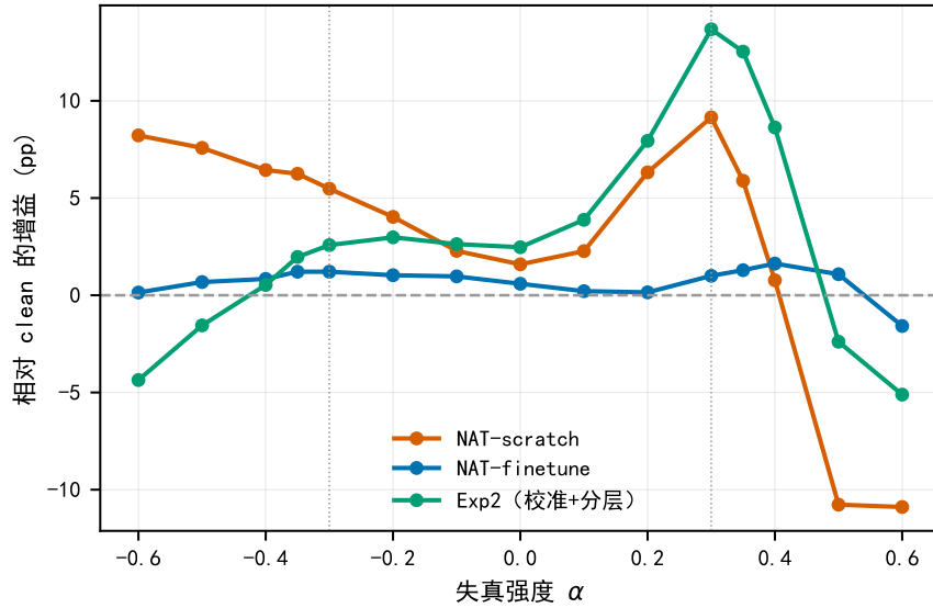
图 6: 非线性感知训练的收益严格限定在训练分布之内 (CIFAR-10 / SimpleCNN)。纵轴为相对同架构干净模型的增益; 竖直虚线标出训练区间 \pm 0.3 。Scratch 策略在正侧外推区迅速归零 ( \alpha = +0.4 时 +0.77 ) 并反转劣势 ( \alpha = +0.5 时 -10.77 )，而负侧保持正值。数据: outputs/extension4_alpha_wide/alpha_wide_scan_summary.csv。
