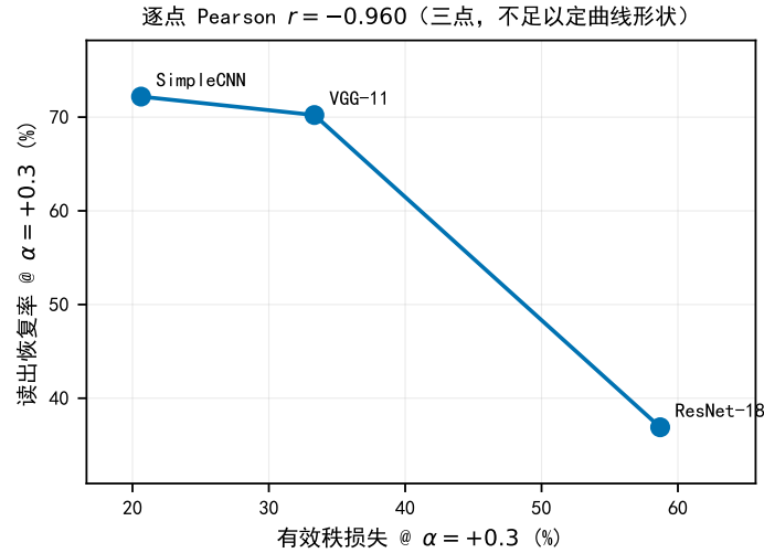
图 7: 秩损失与读出可恢复量的关系 (三点)。恢复率定义为读出适配在 \alpha = +0.3 的精度除以同一读出文件里原始头在 \alpha = 0 的精度。三点在 \alpha = +0.3 上单调, 逐点 Pearson r = -0.960 。三点不足以定曲线形状, 形状提示为”先平后塌”。数据: rank_stats*.csv 与 v3_readout_repair/*ep24*.csv。
