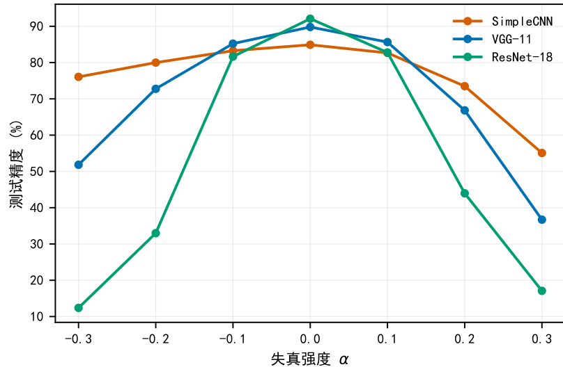
图 1: 任务 1: 三个架构的非线性敏感性 (CIFAR-10)。 \alpha = +0.3 时 SimpleCNN / VGG-11 / ResNet-18 分别跌 29.82 / 53.10 / 75.01 个百分点。数据: outputs/task1_*/alpha_sensitivity.csv。
