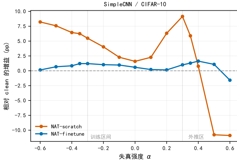
图 5： 非线性感知训练的收益是训练分布内的属性。SimpleCNN 上两种训练策略相对于干净模型的增益沿 \alpha 轴的变化；竖直虚线标出训练区间 \pm 0.3 ，其外为外推区。正侧在 \alpha \approx 0.4 处归零、 \alpha = +0.5 反转为 -10.77 ；负侧在外推区保持正值并略有上升。注意：本图数据集为 CIFAR-10 （干净精度 84.90），与正文其余各图的 CIFAR-100 不同，跨图不可直接比较绝对值。数据：outputs/extension4_alpha_wide/alpha_wide_scan_summary.csv。
