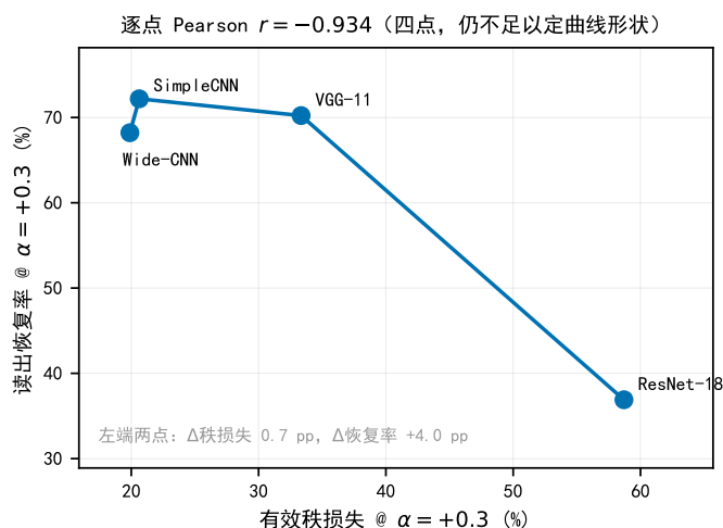
图 10: 秩损失与读出可恢复量 (四点, r = -0.934 )。恢复率 = 读出适配 @ \alpha = +0.3 的精度 \div 同一文件里原始头 @ \alpha = 0 的精度。四点已不是单调关系: 最左两点秩损失只差 0.7 个百分点, 恢复率却差 4.0 个百分点。四点仍不足以定曲线形状: 形状提示为”先平后塌”。
