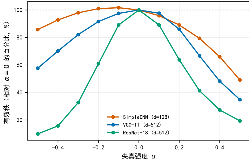
图 9: 正侧失真使末端特征的有效秩塌陷；负侧的形态随主干而异（SimpleCNN 几乎不动，VGG-11 与 ResNet-18 两侧都塌，ResNet-18 的负侧更甚）。纵轴为按各模型 \alpha = 0 归一化的有效秩 \exp(-\sum p_i \ln p_i) ；特征维数分别为 128 / 512 / 512。数据：outputs_cifar100/v5_rank_collapse/rank_stats*.csv。
