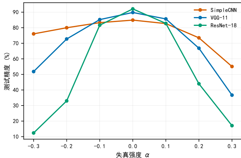
图 1: 任务 1: 三个架构的非线性敏感性 (CIFAR-10)。 \alpha = +0.3 时 SimpleCNN / VGG-11 / ResNet-18 分别跌 29.82 / 53.10 / 75.01 个百分点。数据: outputs/task1_*/alpha_sensitivity.csv。
