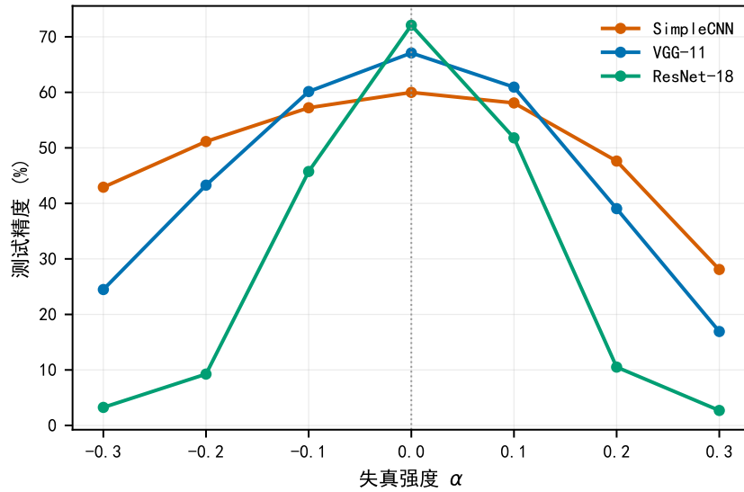
图 5: 失真的方向性与容量依赖 (CIFAR-100)。三个主干在七点上的扫描；正侧跌落大于负侧（该方向在 SimpleCNN 与 VGG-11 上明显，在 ResNet-18 上几乎消失：两侧跌幅 69.39 对 68.84），且随容量与深度单调放大。数据：outputs_cifar100/task1_*/alpha_sensitivity.csv。
