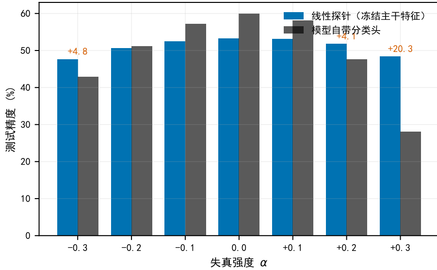
图 6: 探针 headroom: 灾难尾的标签信息仍然线性可达。在同一冻结主干的末端特征上, 线性探针 (实心) 与原始头 (空心, 即模型自带的分类头, 产物里的 a_original_fc ) 的精度; 7 个 \alpha 点, CIFAR-100 全量测试集 (10000 张)、best 权重、单种子。 \alpha = +0.3 时相差 20.26 个百分点; 同样的探针在加性高斯噪声 \sigma = 0.3 下只有 7.50。数据: outputs_cifar100/v7_probe_audit/ra_onprotocol_main.csv 。
