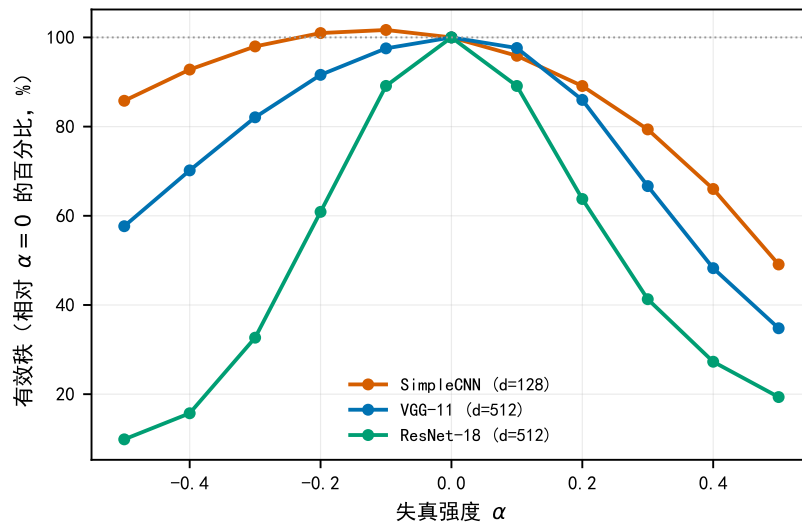
图 9: 正侧失真使末端特征的有效秩塌陷; 负侧的形态随主干而异 (SimpleCNN 几乎不动, VGG-11 与 ResNet-18 两侧都塌, ResNet-18 的负侧更甚)。纵轴为按各模型 \alpha = 0 归一化的有效秩 \exp(-\sum p_i \ln p_i) ; 特征维数分别为 128 / 512 / 512。数据: outputs_cifar100/v5_rank_collapse/rank_stats*.csv。
