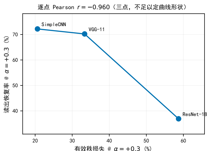
图 10: 秩损失与读出可恢复量 (三点, r = -0.960 )。恢复率 = 读出适配 @ \alpha = +0.3 的精度 \div 同一文件里原始头 @ \alpha = 0 的精度。三点不足以定曲线形状; 形状提示为“先平后塌”。
