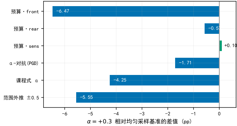
图 8: 训练端的补救路径在 \alpha = +0.3 上没有一条显著优于均匀采样基准 (CIFAR-100 / SimpleCNN)。数据: outputs_cifar100/v3_methods/*/alpha_sensitivity.csv。
