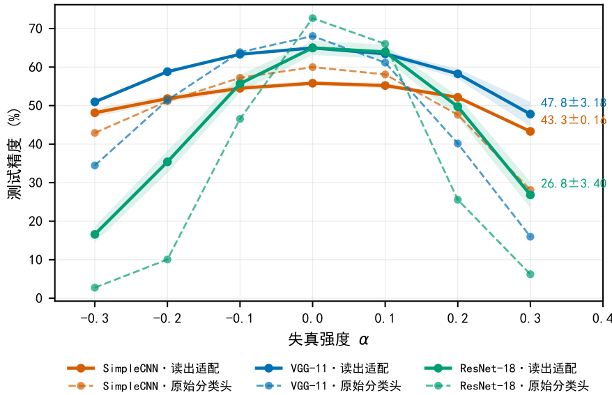
图 7：读出适配跨三个主干一致抬升尾部（CIFAR-100，3 个种子的逐点均值）。实线为读出适配（readout-NAT，主干全冻结，可训练参数占全模型 5.04%/0.55%），虚线为各模型的原始头。数据：outputs_cifar100/v3_readout_repair/*ep24*.csv。
