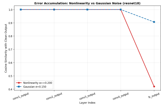
图 21: ResNet-18 非线性与高斯噪声的层误差累积对比
