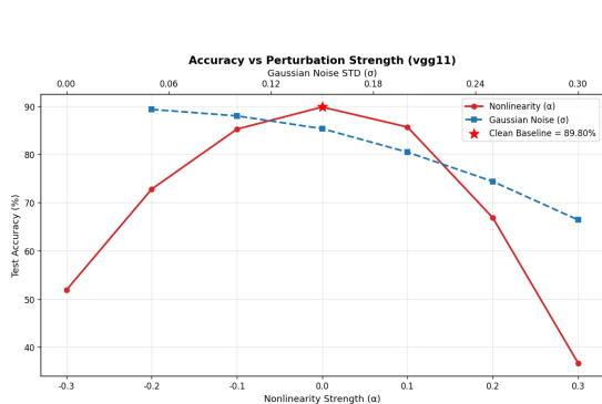
图 18: VGG-11 非线性与高斯噪声精度对比
