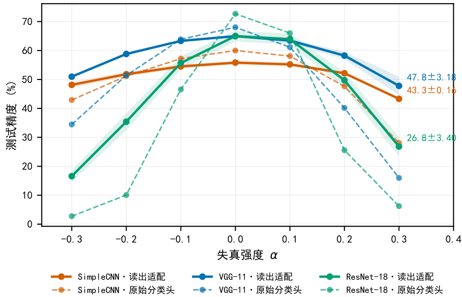
图 3: 读出适配跨三个主干一致抬升尾部。实线为 readout-NAT (冻结主干、只重训线性读出, 可训练参数占全模型 5.04%/0.55%); 每个主干的原始分类头用与该主干同色的虚线; 每个主干为 3 个种子的逐点均值, 阴影为该点上 3 个种子的 \pm 1 总体标准差。α = +0.3 处的标注为均值 \pm 总体标准差。数据: outputs_cifar100/v3_readout_repair/*ep24*.csv。
