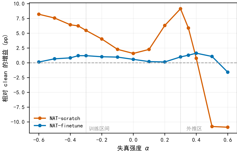
SimpleCNN / CIFAR-10
