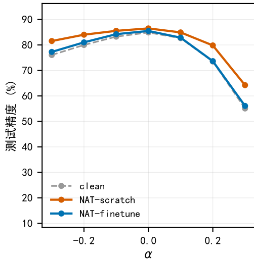
SimpleCNN
