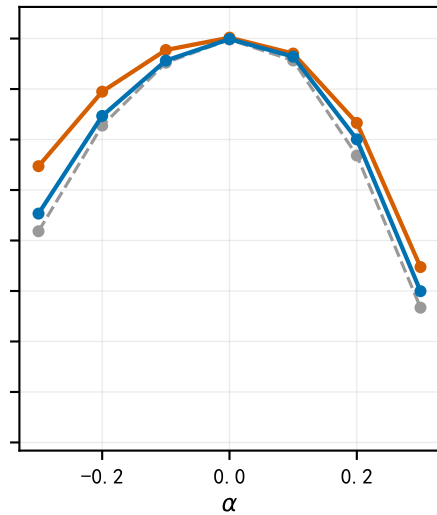
VGG-11
