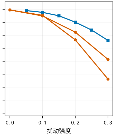
VGG-11
