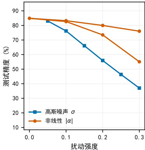
SimpleCNN
