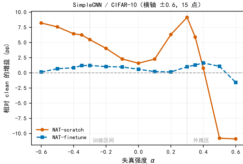
图 5: 非线性感知训练的收益是训练分布内的属性。SimpleCNN 上两种训练策略相对于干净模型的增益沿 \alpha 轴的变化。横轴 \pm 0.6 (15 点), 范围大于正文其余各图的 \pm 0.3 (7 点); 竖直虚线标出训练区间 \pm 0.3 , 其外为外推区。 NAT-scratch (实线圆点): 正侧在 \alpha \approx 0.4 处归零 (+0.77)、 \alpha = +0.5 反转为 -10.77; 负侧在外推区保持正值并略有上升 (-0.4 时 +6.44 \rightarrow -0.6 时 +8.22)。 NAT-finetune (虚线方点): 正侧在整个外推区基本平坦 ( |\Delta| < 1.7 , 到 \alpha = +0.6 才转为 -1.58); 负侧随外推距离缓慢衰减 (+1.21 \rightarrow +0.14)。注意: 本图数据集为 CIFAR-10 (干净精度 84.90), 与正文其余各图的 CIFAR-100 不同, 跨图不可直接比较绝对值。数据: outputs/extension4_alpha_wide/alpha_wide_scan_summary.csv。
