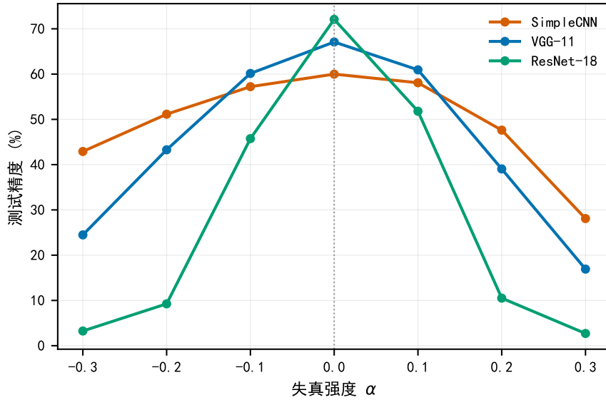
图 1: 失真的方向性与容量依赖。三个主干在 CIFAR-100 上的七点扫描；全量测试集、best 权重、纯推理。正侧 ( \alpha > 0 ) 的跌落大于负侧，但不对称倍率随容量递减： |\alpha| = 0.3 处”正侧跌幅 ÷ 负侧跌幅”在 SimpleCNN / VGG-11 / ResNet-18 上依次为 1.87 / 1.18 / 1.01——方向性在浅层显著，在最深的主干上几乎消失。数据：outputs_cifar100/task1_*/alpha_sensitivity.csv。
