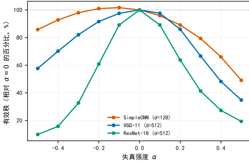
图 6: 失真使末端特征的有效秩塌陷, 但两侧的形态按主干分化。纵轴为按各模型 \alpha = 0 归一化后的有效秩 ( \exp(-\sum p_i \ln p_i) , p_i 为归一化奇异值); 横轴 11 个 \alpha 点。三个主干的特征维数分别为 128 / 512 / 512。 \alpha = \pm 0.3 处的秩损失分别为 20.6% / 2.0% (SimpleCNN)、33.3% / 17.9% (VGG-11)、58.7% / 67.3% (ResNet-18)——“负侧”几乎不动”只在浅层的 SimpleCNN 上成立; ResNet-18 的负侧比正侧掉得更多。数据: outputs_cifar100/v5_rank_collapse/rank_stats*.csv。
