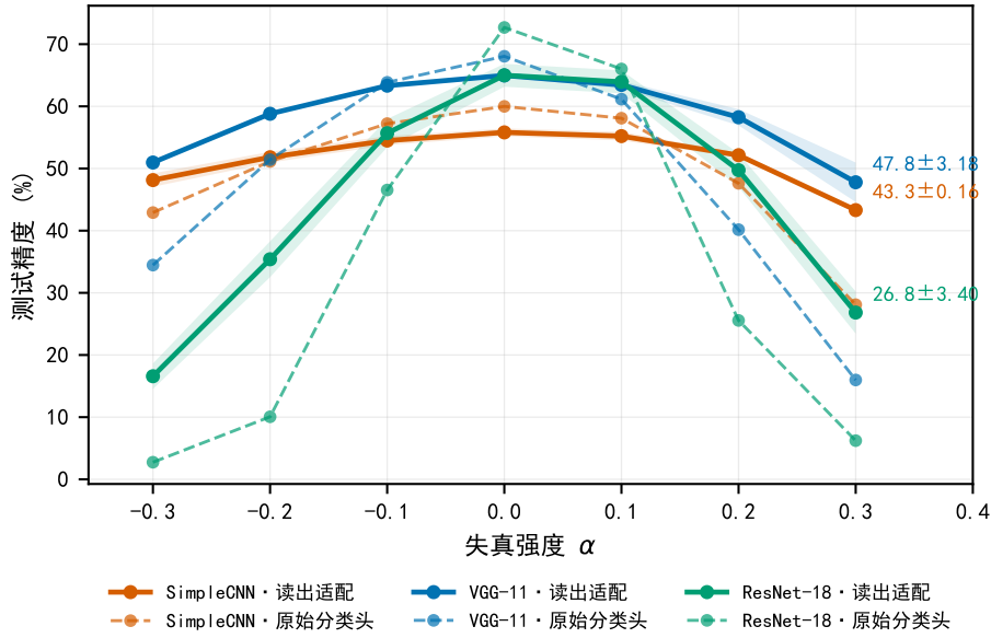
图 3: 读出适配跨三个主干一致抬升尾部。实线为 readout-NAT (冻结主干、只重训线性读出, 可训练参数占全模型 5.04%/0.55%); 每个主干的原始分类头用与该主干同色的虚线; 每个主干为 3 个种子的逐点均值, 阴影为该点上 3 个种子的 \pm 1 总体标准差。 \alpha = +0.3 处的标注为均值 \pm 总体标准差。数据: outputs_cifar100/v3_readout_repair/*ep24*.csv。
