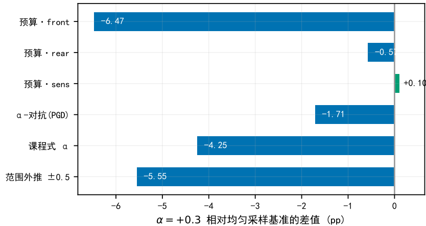
图 4: 训练端的补救路径在 \alpha = +0.3 上没有一条显著优于均匀采样基准（最好的一条为 +0.10 pp）。差值以基准（均匀采样， \alpha = +0.3 时 26.03%）为零线；绿 = 高于基准、蓝 = 低于基准；预算分配三种轮廓、 \alpha 空间对抗训练（PGD）、课程式采样、训练范围外推至 \pm 0.5 。CIFAR-100 / SimpleCNN / 120 epoch / 单种子。数据：outputs_cifar100/v3_methods/*/alpha_sensitivity.csv。
