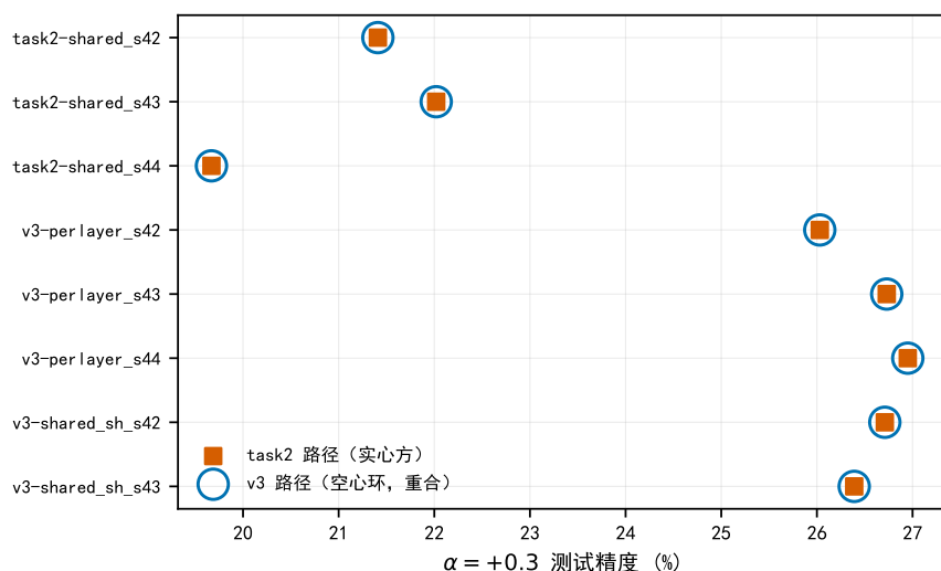
图 11: 交叉评估: 差异不在评估路径。把 8 个权重分别在另一脚本原样导入的评估函数下重扫, 两条路径给出逐位相同的读数 (含干净精度) —— (图中每条读数由重合的两枚标记表示: 实心方 = task2 路径、空心环 = v3 路径; 两者逐位相同故完全重合); 但两组权重稳定分成两簇 (A 脚本 19.7~22.0, B 脚本 26.0~27.0)。数据: outputs_cifar100/v6_p4e_crosspath/crosspath.csv 。
