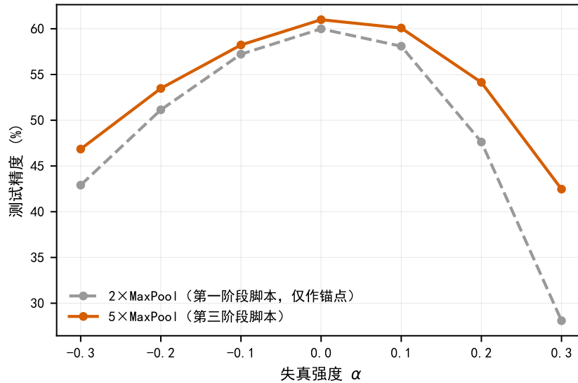
图 8: 池化密度是独立的架构级杠杆。把 SimpleCNN 的最大池化层从 2 个增加到 5 个——参数量不变、训练成本为零。同协议同 seed 配对 (120 epoch、逐层独立采样) 的读数是 \alpha = +0.3 从 26.03 提升到 41.55 (+15.52, 各单 seed)。图中灰色虚线为第一阶段脚本的产物, 与实线的 v3_methods 分属两个阶段、不同协议, 仅作参考点、不参与任何同协议对比 (正文若引用 28.09 \rightarrow 42.47, 即横跨这两条曲线, 须显式注明其跨协议性; 该臂自身三个同协议种子的均值为 40.29 \pm 1.58 , 见正文)。数据: outputs_cifar100/v3_methods/simple_cnn_mp_clean_uniform/alpha_sensitivity.csv 与 task1_simplecnn/alpha_sensitivity.csv。
