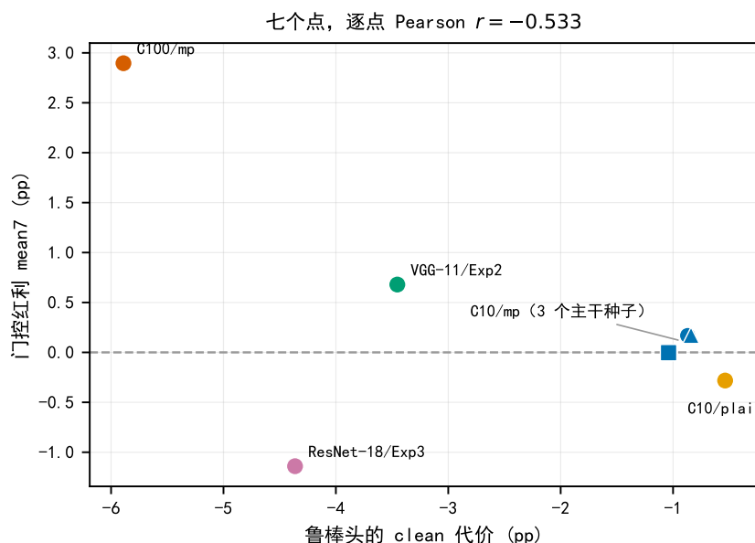
图 9: 门控红利不随鲁棒头代价单调增长。横轴为鲁棒头相对干净头在 \alpha = 0 的精度损失（负值 = 鲁棒头更差），纵轴为门控相对单用鲁棒头在 mean7 上的增益。七个点取自四个主干配置与两个数据集，各 3 个种子。（C10/mp 的三个主干种子在图中以三种标记画出、共用同一标签。）逐点 Pearson r = -0.533 ；去掉 CIFAR-100 远点后 n = 6 时符号反转为 +0.351 。数据：v5_full_recipe/recipe*.csv。
