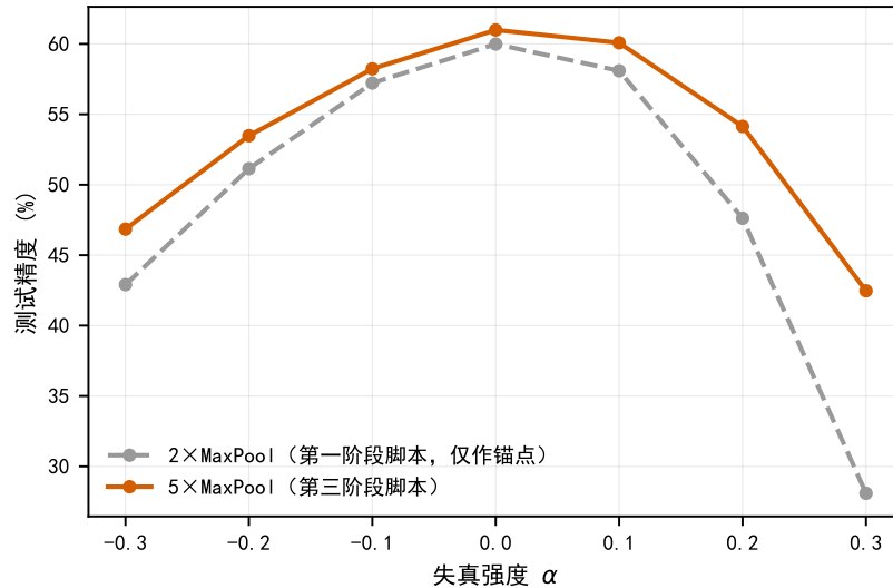
图 11: 池化密度是零训练成本的独立架构杠杆。MaxPool 从 2 个加到 5 个 (参数量不变、训练脚本不变): \alpha = +0.3 从 28.09 到 42.47。虚线为第一阶段脚本的产物: 它与实线出自不同训练脚本 (本项目实测跨脚本的精度数字不可直接比较), 故属异协议、仅作参考点, 不与实线并列比较。
