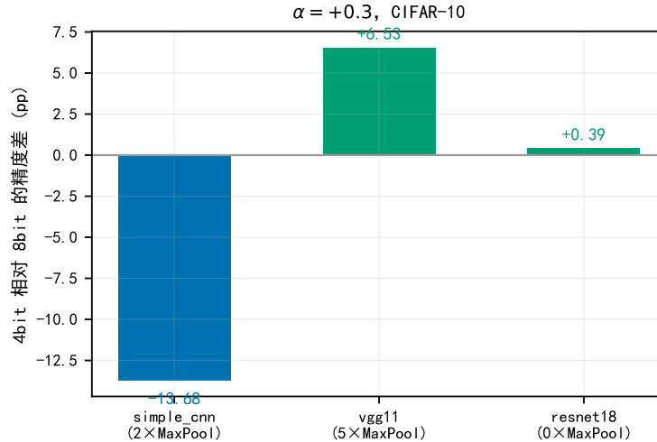
图 7: Dithering 增益的架构依赖 (CIFAR-10, \alpha = +0.3 )。横轴上标注每个架构的 MaxPool 数量。增益与 MaxPool 密度同向但要足够密——2 个 MaxPool 的 SimpleCNN 是负增益，0 个的 ResNet-18 无效应。数据: outputs/extension5_dithering_vgg11/arch_dithering_summary.csv。
