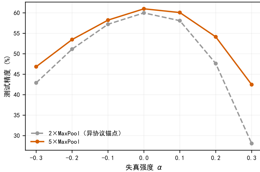
图 8: 池化密度是独立的架构级杠杆。把 SimpleCNN 的最大池化层从 2 个增加到 5 个——参数量不变、训练脚本不变、训练成本为零—— \alpha = +0.3 从 28.09 提升到 42.47。虚线为第一阶段 100 epoch 的产物, 与实线的 120 epoch 不同协议, 仅作参考点、不参与同协议对比。数据: outputs_cifar100/v3_methods/simple_cnn_mp_clean_uniform/alpha_sensitivity.csv。
