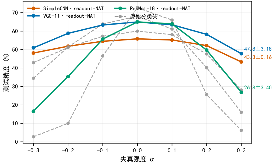
图 3: 读出适配跨三个主干一致抬升尾部。实线为 readout-NAT (冻结主干、只重训线性读出, 可训练参数占全模型 5.04%/0.55%), 虚线为各模型自带的分类头; 每个主干为 3 个种子的逐点均值。 \alpha = +0.3 处的标注为均值 \pm 总体标准差。数据: outputs_cifar100/v3_readout_repair/*ep24*.csv 。
