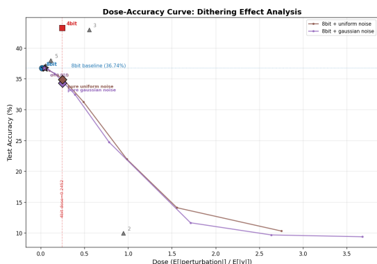
图 30: 噪声剂量-精度曲线: 注入噪声单调下降, 无倒 U 形响应
