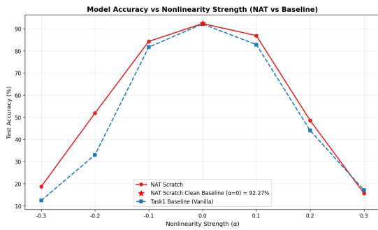
图 11: ResNet-18 NAT-Scratch 与干净基线精度对比
