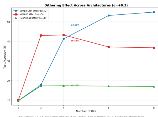
图 31: 三架构 bits-精度对比 (MaxPool 数 0/2/5)
