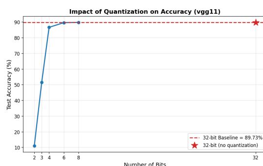
图 23: VGG-11 单独量化精度曲线
