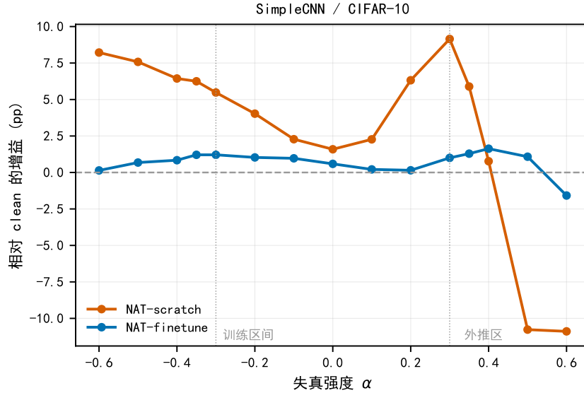
图 5：非线性感知训练的收益是训练分布内的属性。SimpleCNN 上两种训练策略相对干净模型的增益沿 \alpha 轴的变化；竖直虚线标出训练区间 \pm 0.3 ，其外为外推区。正侧在 \alpha \approx 0.4 处归零、 \alpha = +0.5 反转为 -10.77 ；负侧在外推区保持正值并略有上升。注意：本图数据集为 CIFAR-10 （干净精度 84.90），与正文其余各图的 CIFAR-100 不同，跨图不可直接比较绝对值。数据：outputs/extension4_alpha_wide/alpha_wide_scan_summary.csv。
